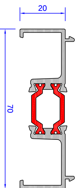
DV559 20mm Add-On
